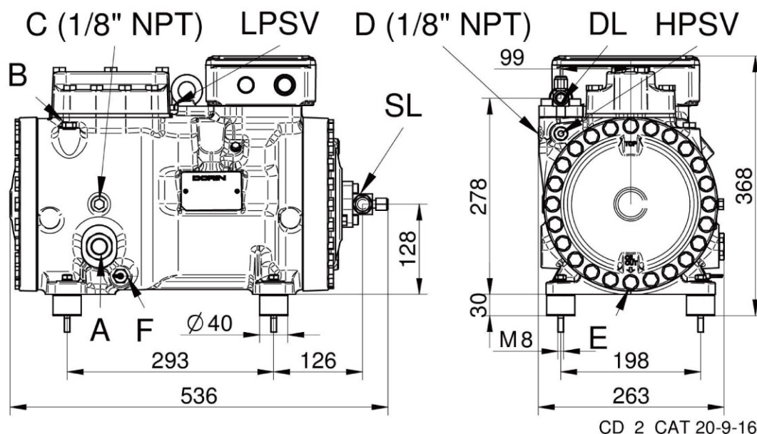
Figure / 外形尺寸
